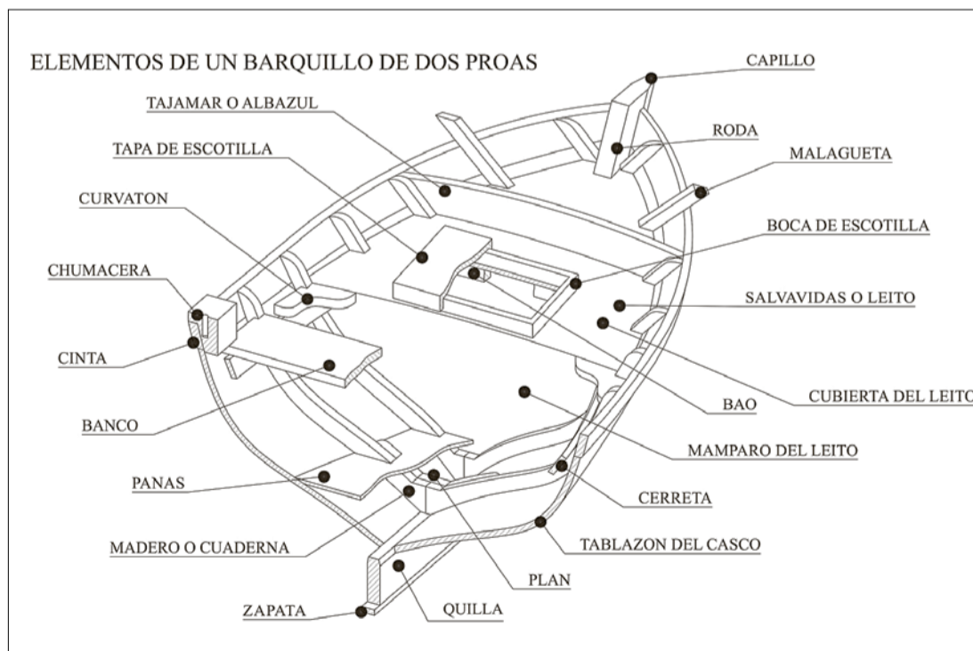
Elementos constructivos del barquillo canario. Imagen cedida y realizada por Daniel Rodríguez Zaragoza.
